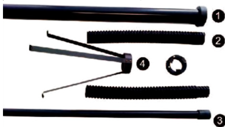
Детали магнитного экстензометра
