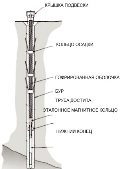
Установка магнитного экстензометра
