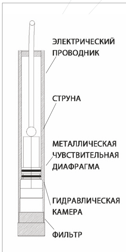
Детали конструкции
